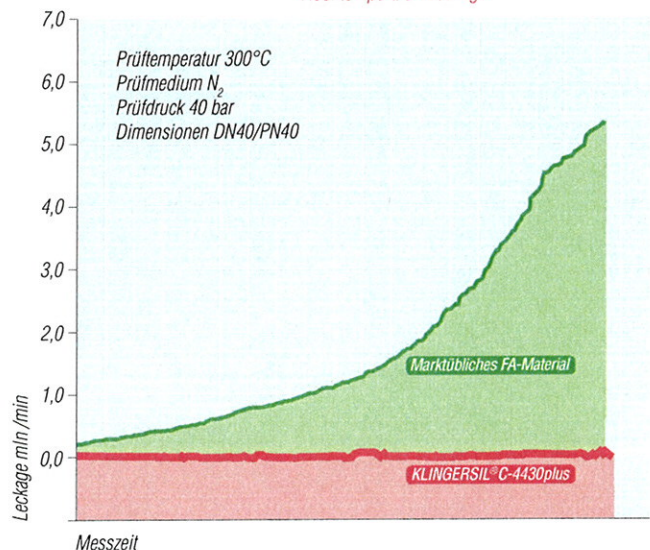
Hochtemperatur-Leckage
