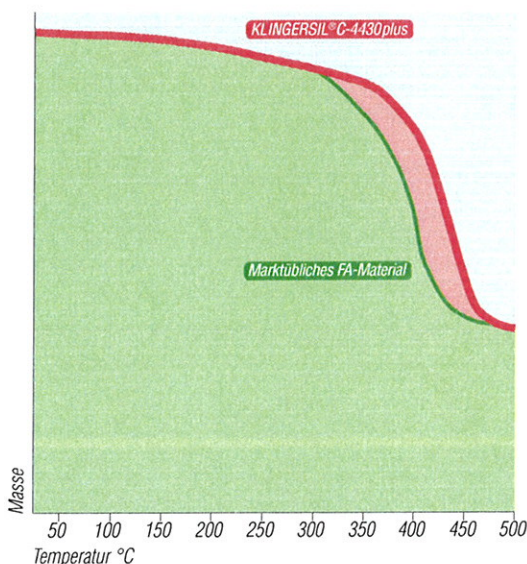
Thermogravimetrische Analyse
