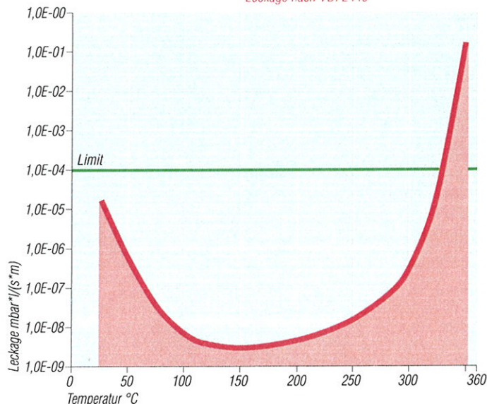
Leckage nach VDI 2440
